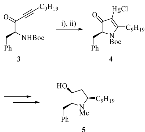
Scheme 1. i) \text{Hg}(\text{OAc})_2 , ii) \text{NaCl} .
